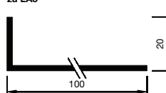
Winkelprofil zu LA3
