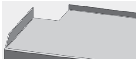
Pfostenklinkung 2-seitig ohne Bord
