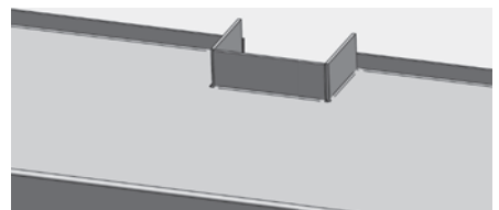
Pfostenklinkung 3-seitig mit Bord
