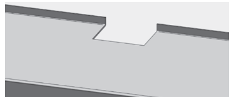
Pfostenklinkung 3-seitig ohne Bord
